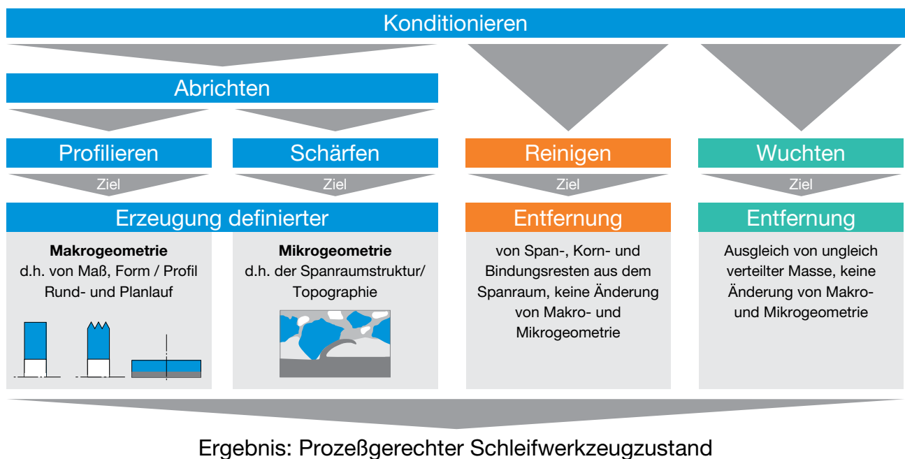
Abbildung 1: Konditionieren - Prozessschritte
