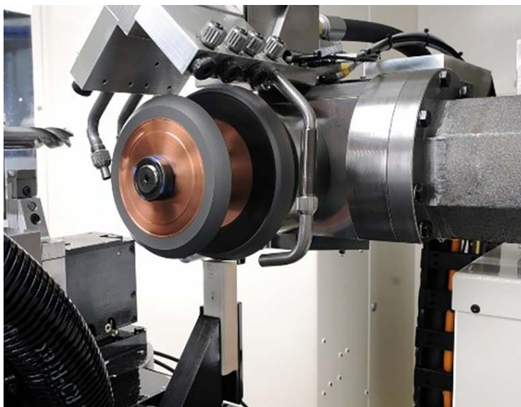
Abbildung 12: Schärfen Diamantschleifscheibe
