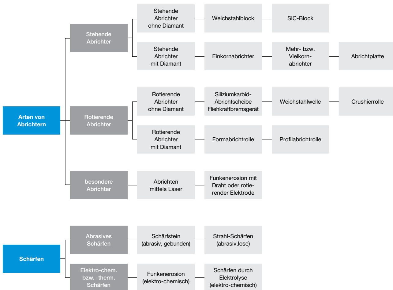
Abbildung 2: Übersicht Abricht- und Schärfverfahren
