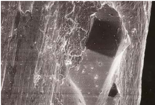
Abbildung 14: Optimale Kornfreistellung/ Kornabstützung
